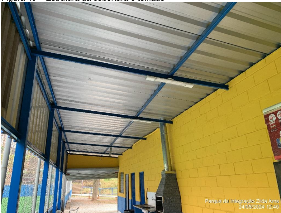
Figura 49 – Estrutura da cobertura e telhado
