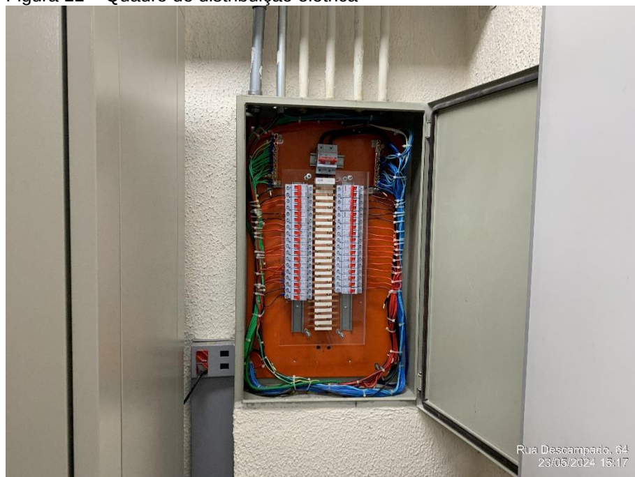
Figura 11 – Quadro de distribuição elétrica
