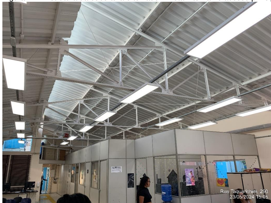
Figura 21 – Estrutura da cobertura e telhado – vista interna no acesso principal
