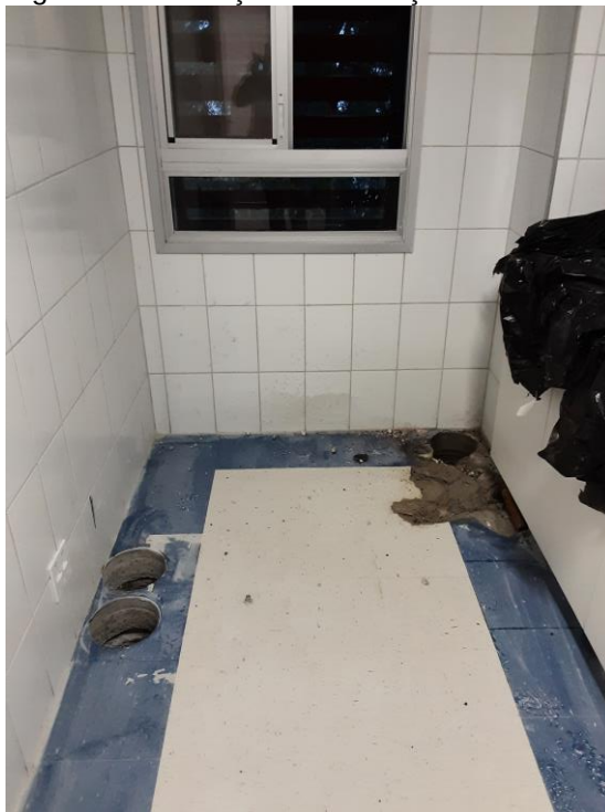
Figura 93 – Serviços de tubulação a realizar.
