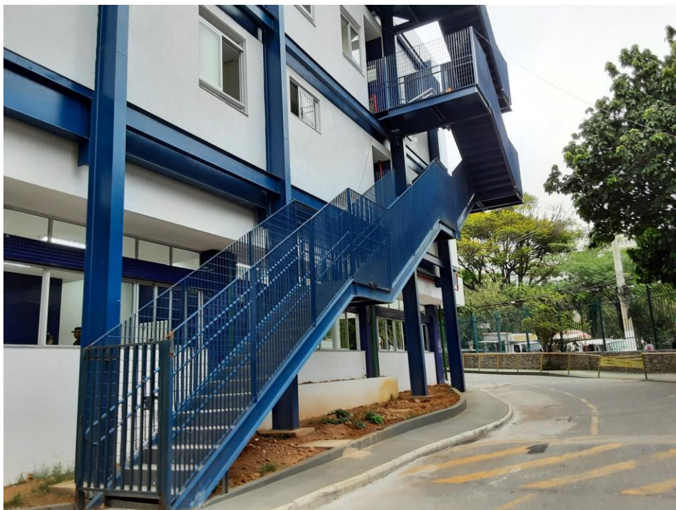
Figura 7 - Vista da escada e estruturas metálicas.
