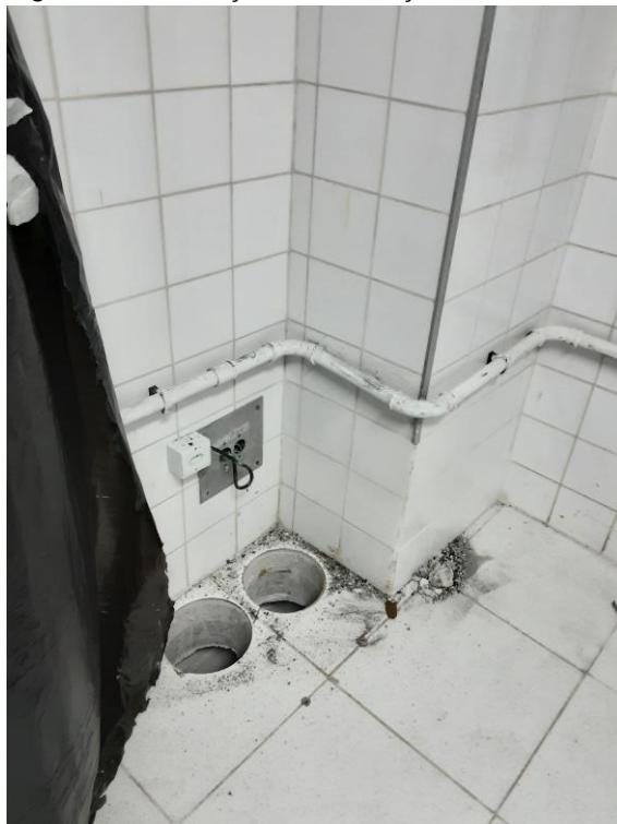
Figura 92 – Serviços de tubulação a realizar.
